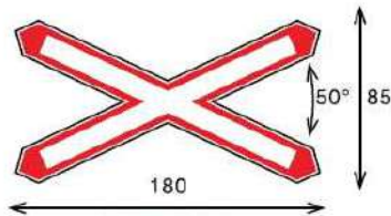
FIG. 10/a CROCE DI S. ANDREA obbligatorio in pellicola classe II
