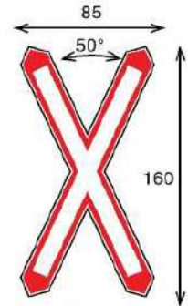
FIG. 10/c CROCE DI S. ANDREA INSTALLATA VERTICALMENTE obbligatorio in pellicola classe II
