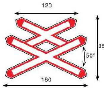
FIG. 10/b DOPPIA CROCE DI S. ANDREA obbligatorio in pellicola classe II
