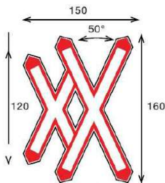
FIG. 10/d DOPPIA CROCE DI S. ANDREA INSTALLATA VERTICALMENTE obbligatorio in pellicola classe II
